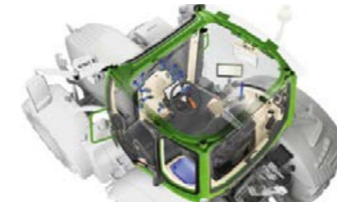
Das ausgeklügelte Belüftungs- und Klimatisierungskonzept bietet eine optimierte Luftverteilung über den Lenkturm und eine Seitendüse für die rechte Scheibe. Dazu kommen eine Überdruckfunktion und die Defrostautomatik. Die Innenraumtemperatur wird im Dashboard angezeigt. Die klappbare Dachluke sorgt für zugfreie Belüftung.
